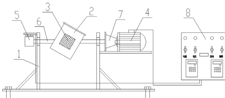
1 外框架 2 料筒 3 电磁振动片 4 电机 5 碳刷 6 旋转轴 7 调速器 8 控制箱
