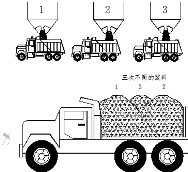
图 6.4.2 混合料前、后、中三次装料示意图
