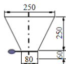
漏斗结构尺寸
