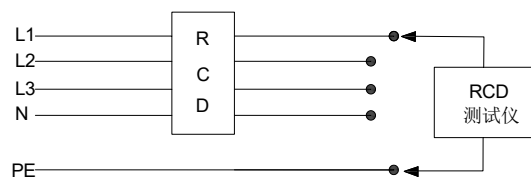
图 1 测试方法
