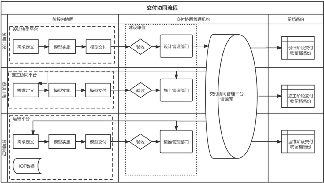
图 6.2.1 交付协同流程图
